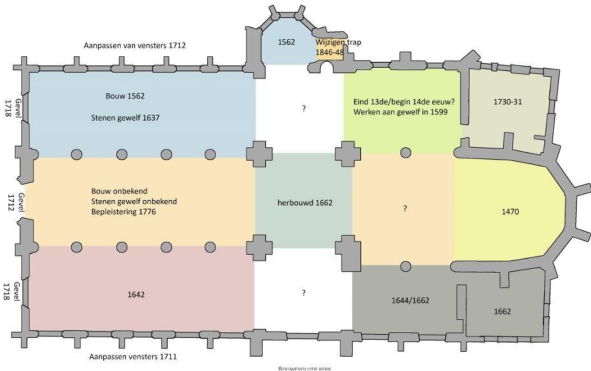
Grafische weergave van de bouwgeschiedenis (p 12 Afb. 1.2. bijlage 8 Stratigrafisch en materiaaltechnisch vooronderzoek O.L.V.-Geboortekerk te Lebbeke, Ornament, 2016, deel 1 (Corpus) en deel 2 (Bijlagen)
